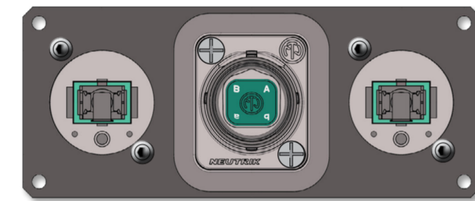
SC OPTI QUAD SC MM
